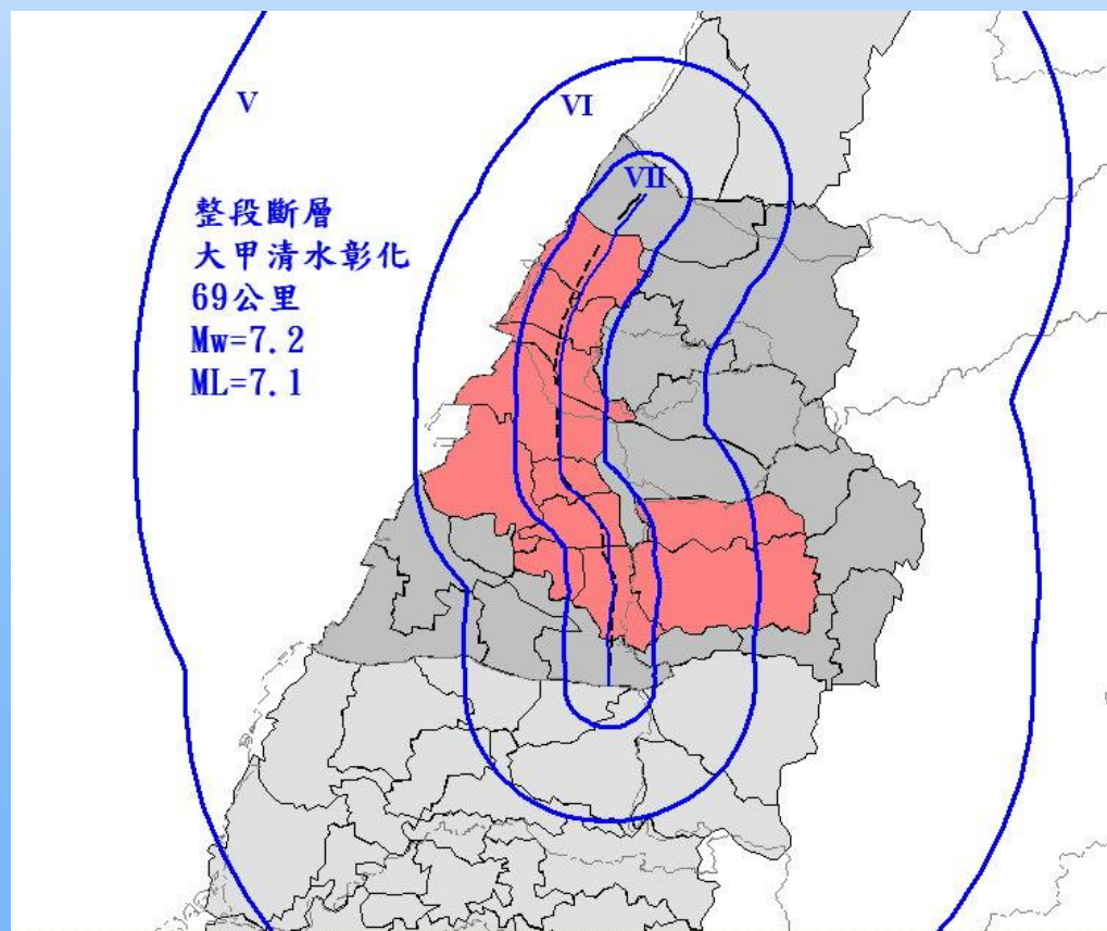
整段斷層(大甲,清水,彰化)地震等震度模擬圖 長度69公里 ML=7.1 深度10公里
