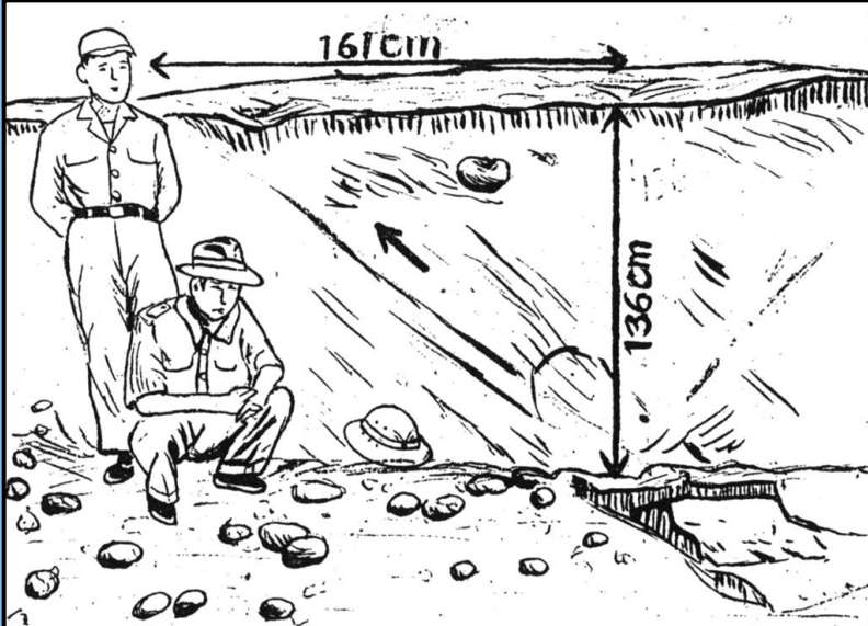
花蓮縣瑞穗鄉富興村之玉里地震斷層露頭
