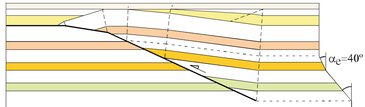
Simple Shear Fault-bend Fold
