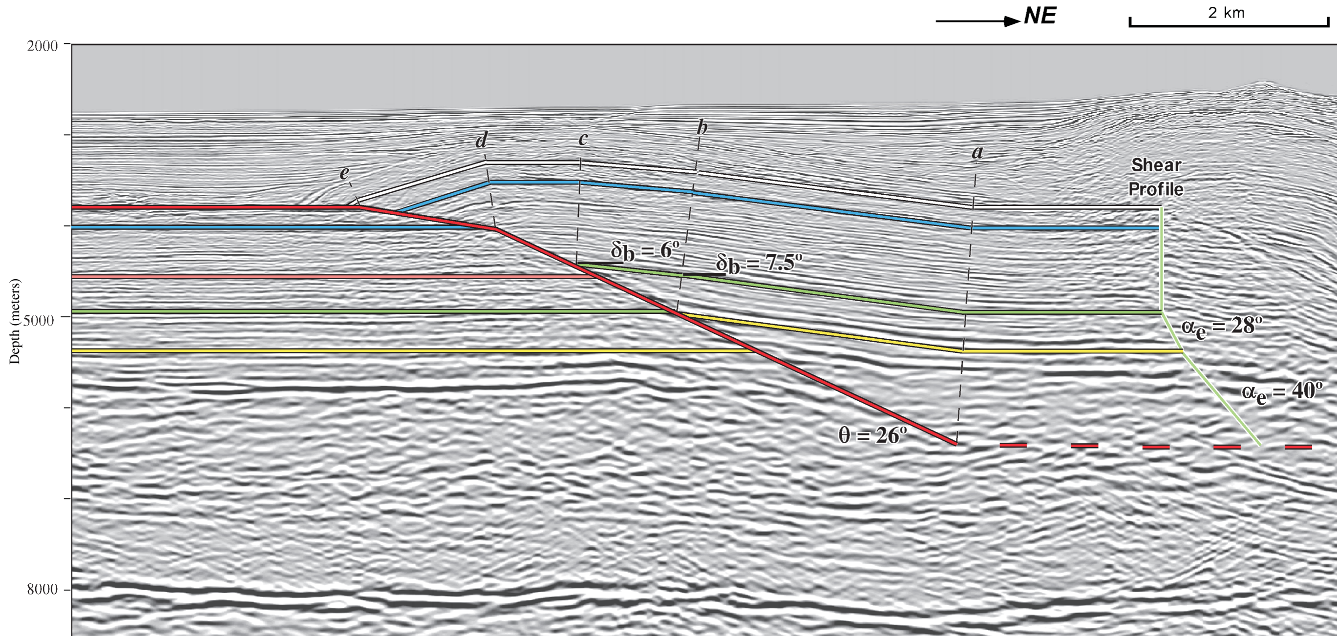
Simple Shear Fault-bend Fold
